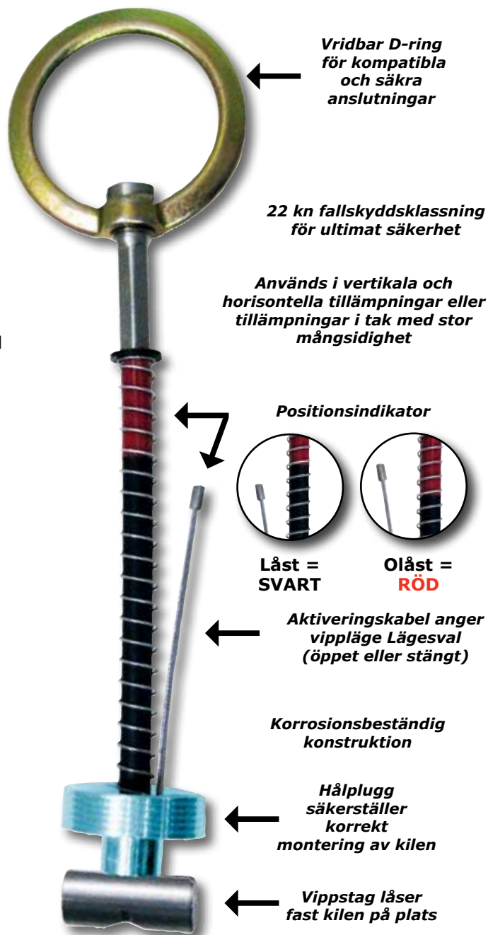
Saflok® förankringsmodell med betongkil: 2100103: Saflok® Expanderankare
